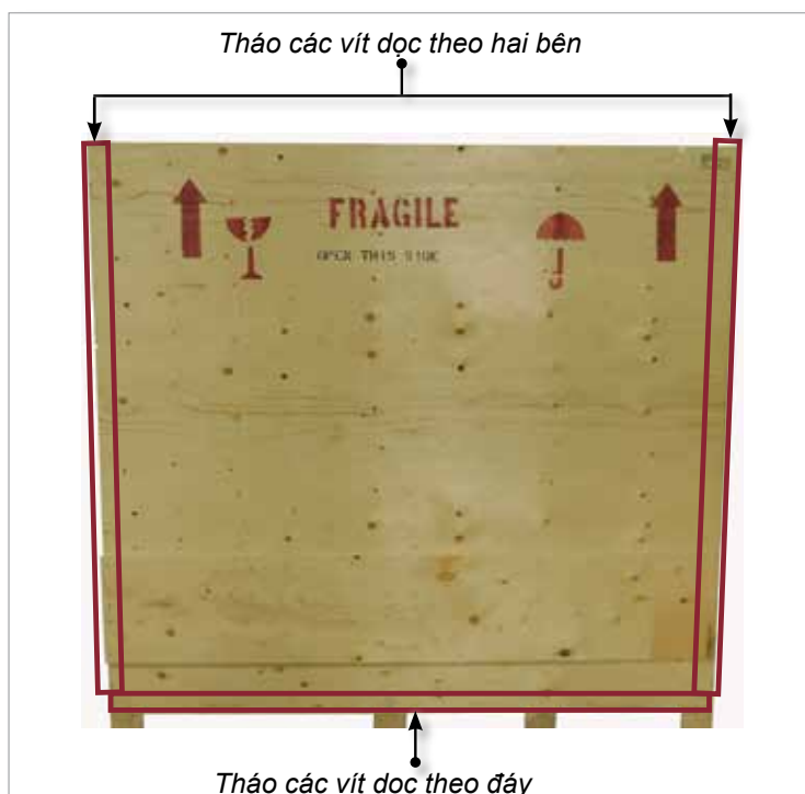
Hình 3-8 Tháo các vít khỏi phía bên và đáy
