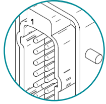
Stecker (M/F) 24-polig Doppelverriegelung
