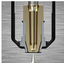
Bi-M C-Sprue
