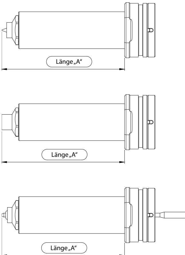
Abbildung 3 Düsenmaße
